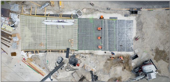
Abb. 7: Gleistragplattenbewehrung der Straßenbahn in München
