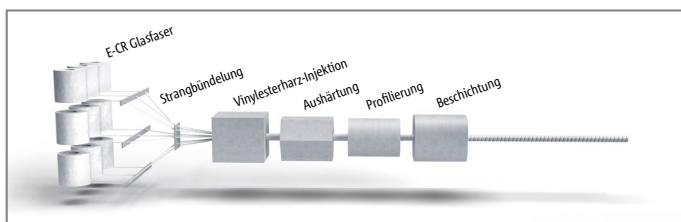
Abb. 2: Im Pultrusionsverfahren zur Herstellung von Combar® werden Glasfasern dicht gebündelt, durch ein Werkzeug gezogen und mit flüssigem Kunstharz umschlossen. Anschließend werden die Stäbe profiliert.
