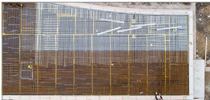
Abb. 8: Bewehrung der Schallschutzmaßnahmen an den vier Weichen der Stadtbahnlinie U72 in Ratingen
